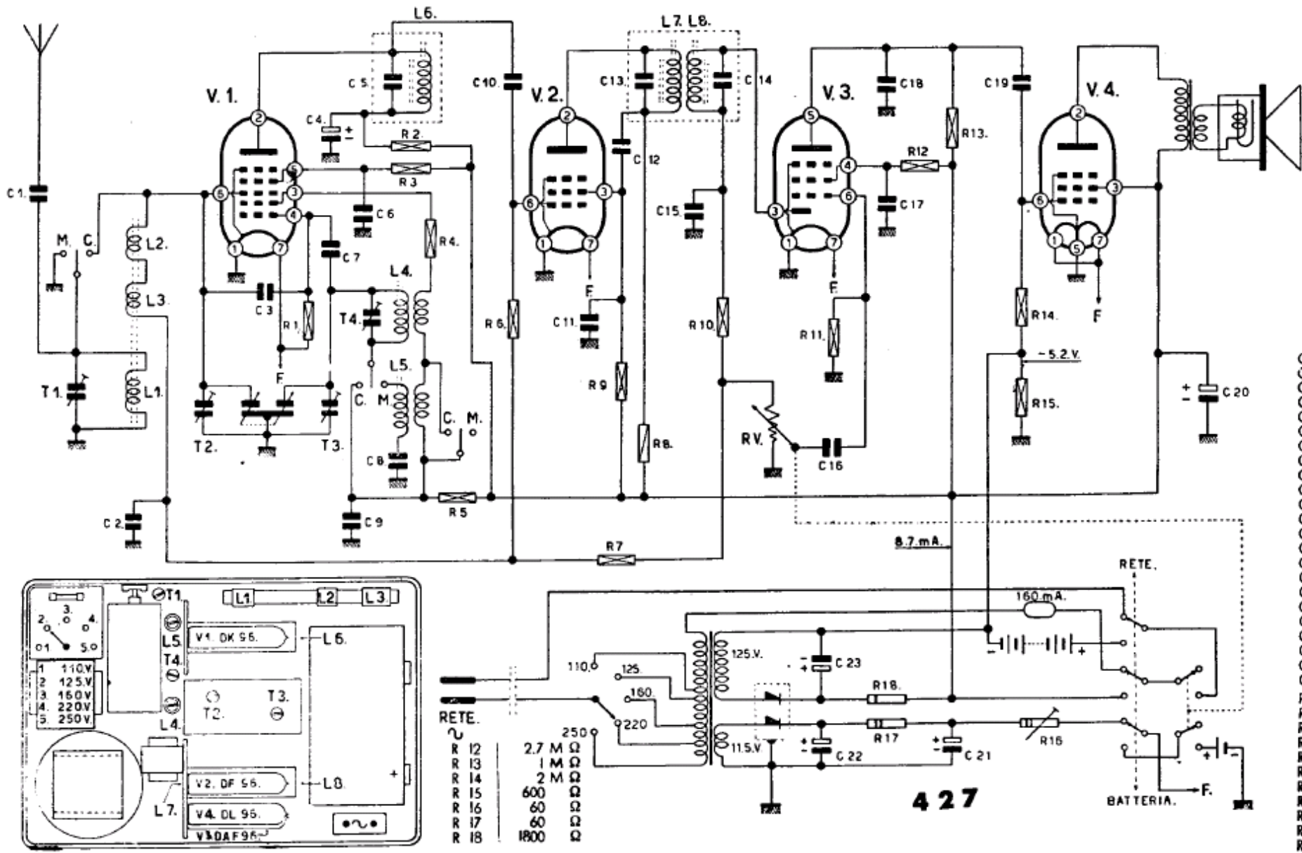
FIMI S.A. - PHONOLA - Mod. 427 trasportabile CC e CA. Una gamma onde medie da 185 a 582 m., una gamma onde corte da 21,4 a 52 m. Media frequenza 468 kc/s. Potenza indistorta 0,2 watt con alimentazione in CA. DK96: pl. 70 V, sc. 68 V, gr. oscillatrice 37 V. DF96: pl. 61 V, sc. 53 V. DAF96: pl. 20 V, sc. 18 V. DL96: pl. 82 V, sc. 85 V.
